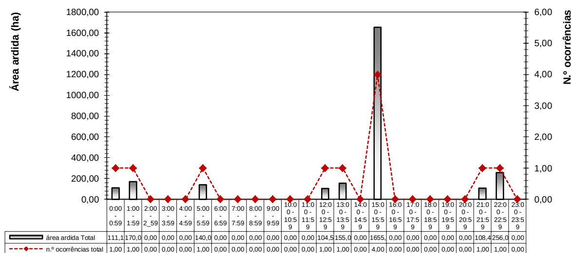
Figura 20 - Distribuição horária da área ardida e n.º de ocorrências dos grandes incêndios 1995-2014, no concelho de Oliveira de Azeméis (ICNF, 2015).
