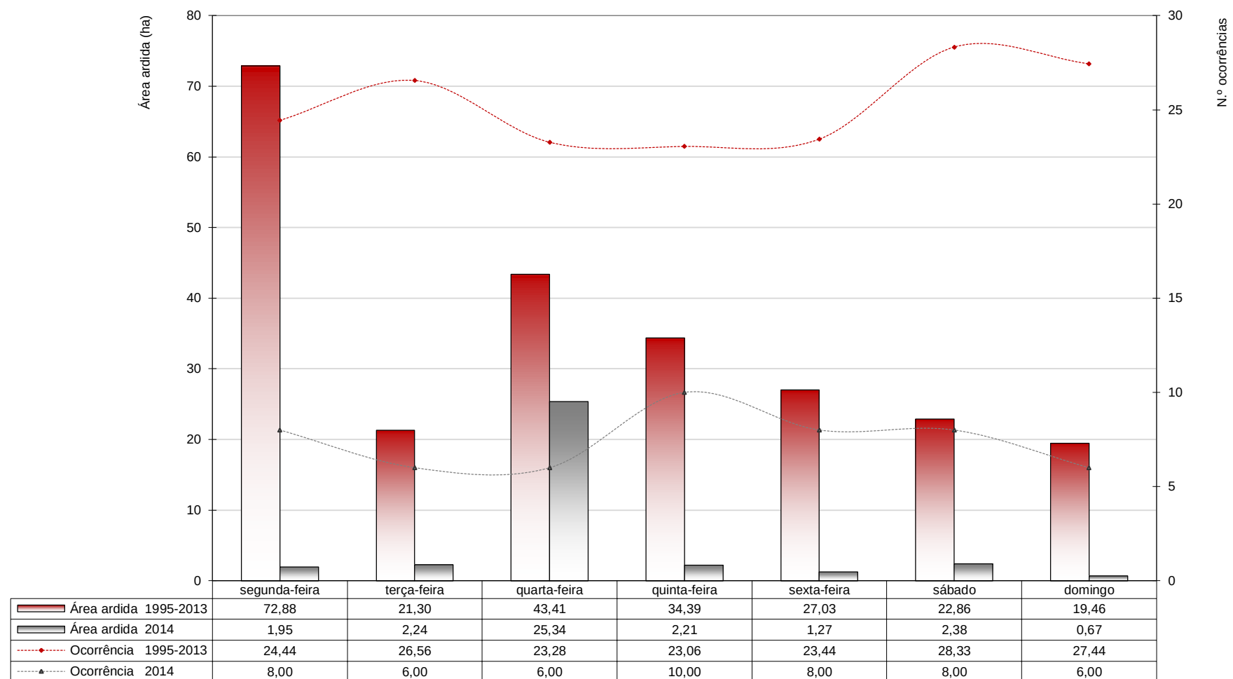
Figura 9 - Distribuição semanal da área ardida e do n.º de ocorrências em 2014 e média 1995-2013, no concelho de Oliveira de Azeméis (ICNF, 2015).
