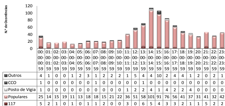
Figura 15 - Distribuição do n.º de ocorrências por fonte de alerta (2007-2014), no concelho de Oliveira de Azeméis (ICNF, 2015).
