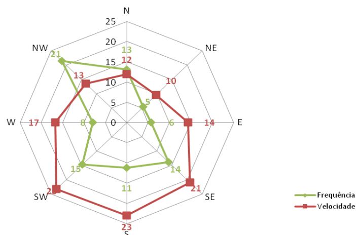
Figura 4 – Padrões eólicos para o concelho de Oliveira de Azeméis (INMG, 1988).
