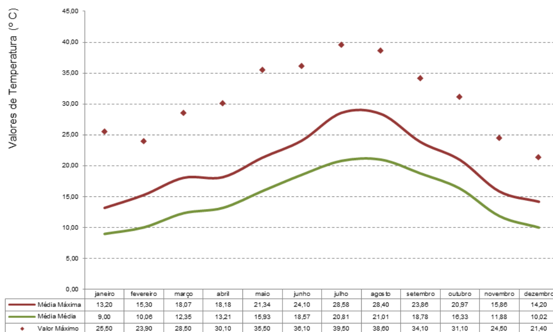
Figura 1 - Valores mensais de temperatura média, média dos valores máximos e valores máximos registados para o período de 1983-2013 (estação meteorológica da Barragem de Burgães) (SNIRH/APA, 2014).
