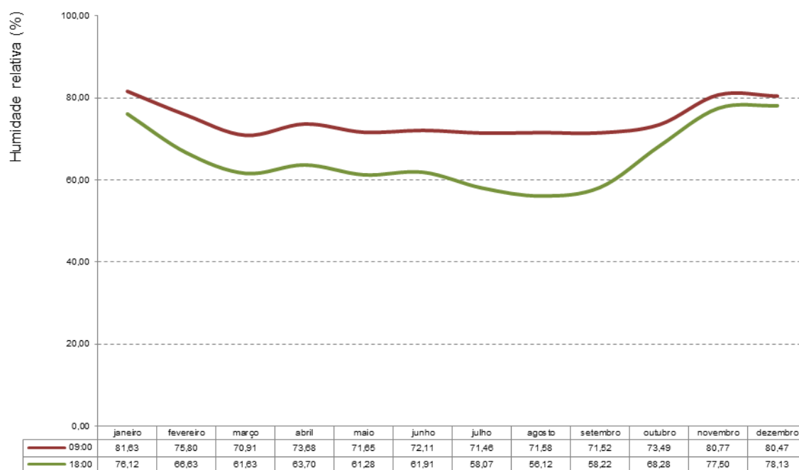
Figura 2 - Valores médios mensais de humidade relativa às 9:00 e às 18:00 (2005-2013) (estação meteorológica da Barragem de Burgães) (SNIRH/APA, 2014).
