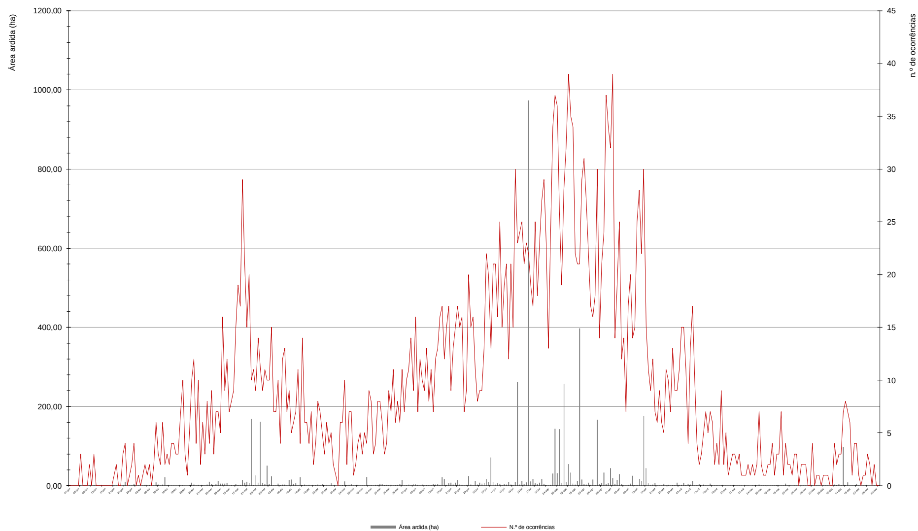
Figura 10 - Valores diários acumulados da área ardida e n.º de ocorrências (1995 a 2014), no concelho de Oliveira de Azeméis (ICNF, 2015).
