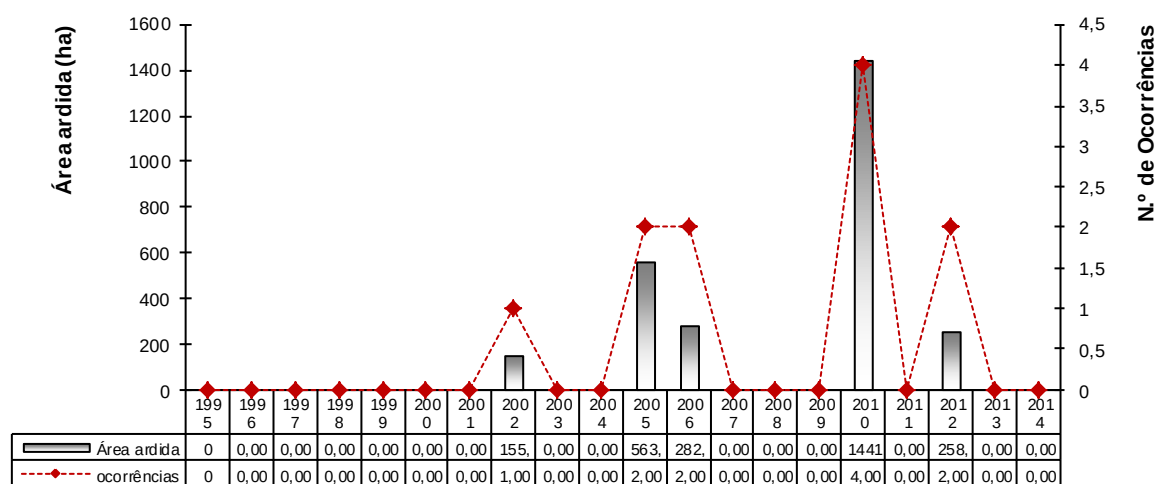
Figura 17 - Distribuição anual da área ardida e n.º de ocorrências dos grandes incêndios 1995-2014, no concelho de Oliveira de Azeméis (ICNF, 2015).
