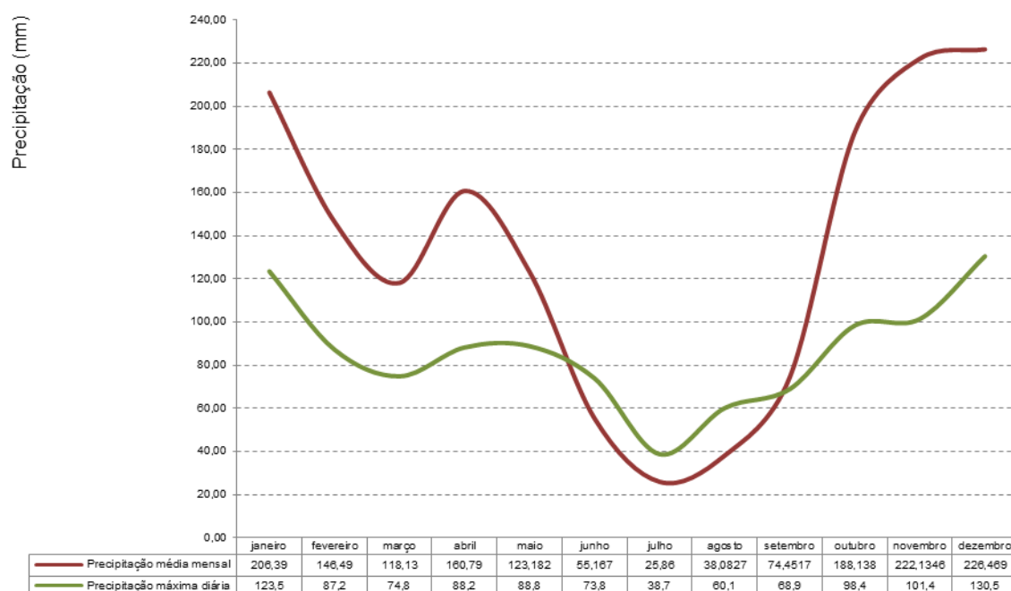
Figura 3 - Valores de precipitação média mensal e máxima diária no concelho de Oliveira de Azeméis (estação meteorológica da Barragem de Burgães) (SNIRH/APA, 2014).
