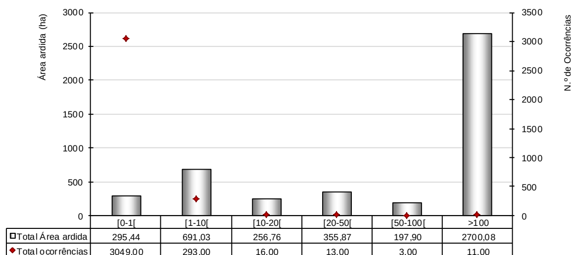
Figura 13 - Distribuição da área ardida e n.º de ocorrências por classes de extensão 1996 – 2014, no concelho de Oliveira de Azeméis (ICNF, 2015).
