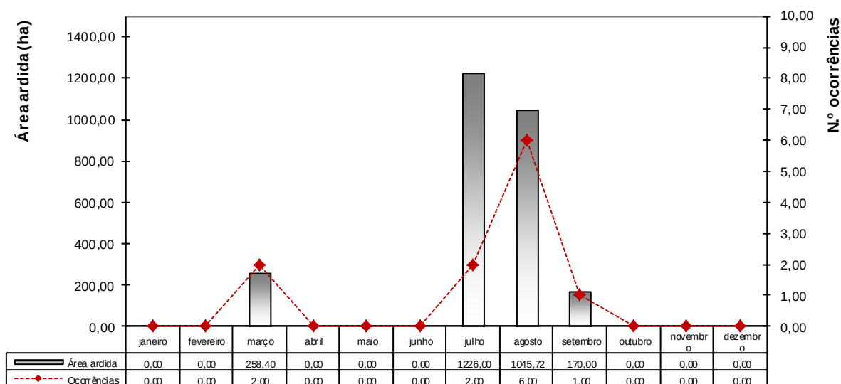
Figura 18 - Distribuição mensal da área ardida e n.º de ocorrências dos grandes incêndios 1995-2014, no concelho de Oliveira de Azeméis (ICNF, 2015).
