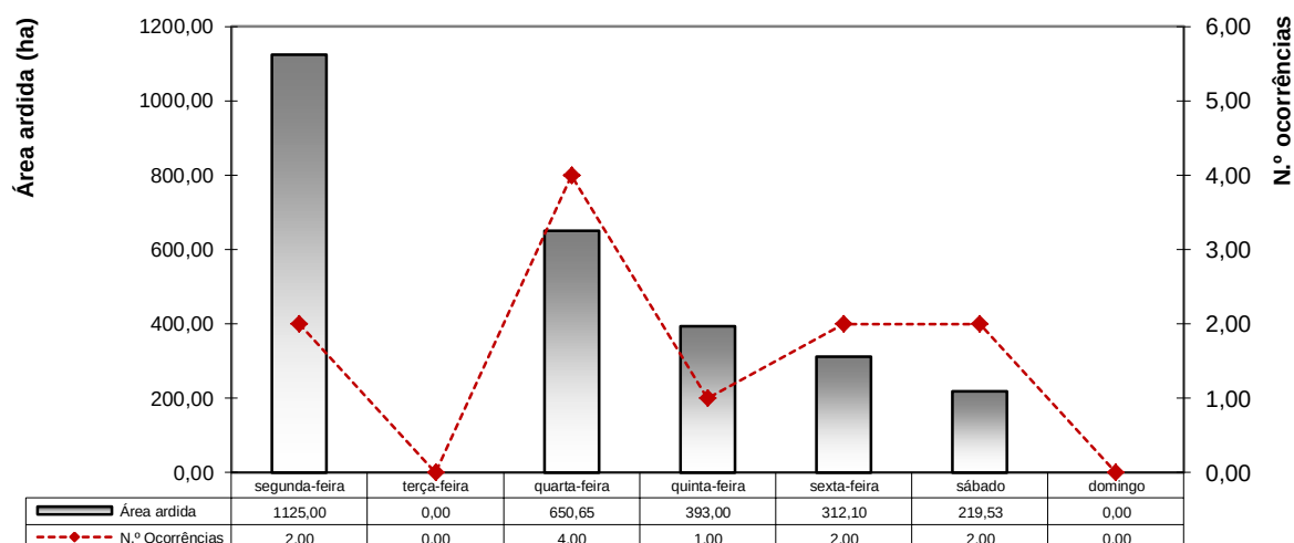
Figura 19 - Distribuição semanal da área ardida e n.º de ocorrências dos grandes incêndios 1995-2014, no concelho de Oliveira de Azeméis (ICNF, 2015).
