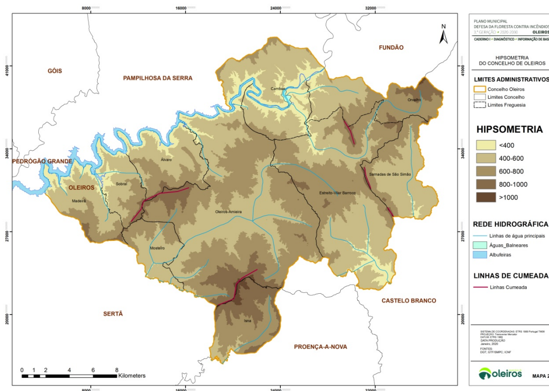
Mapa 2: Hipsometria do concelho de Oleiros
