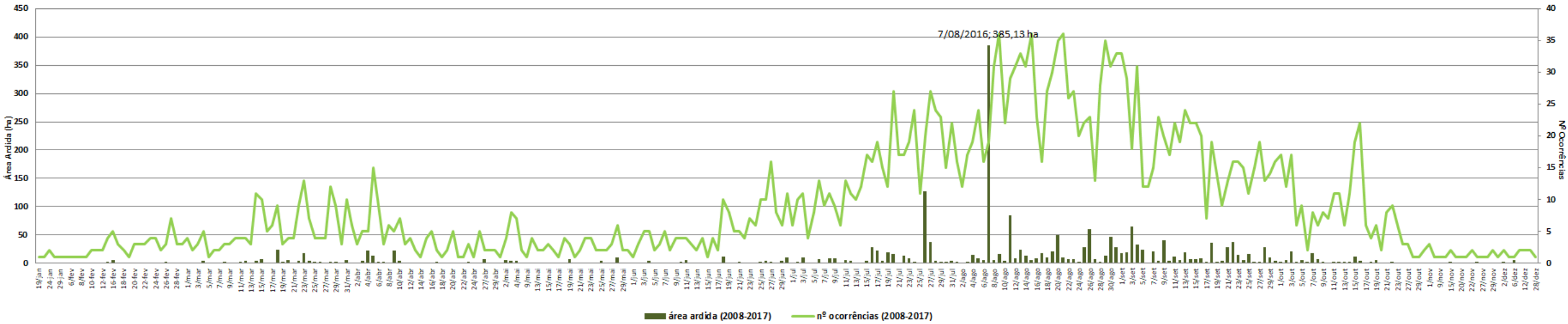
Gráfico 13: Área ardida e número de ocorrências (2008-2017) – distribuição diária
