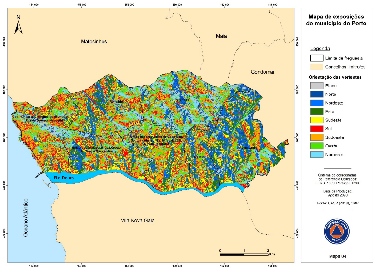
Mapa 4 | Exposição de vertentes
