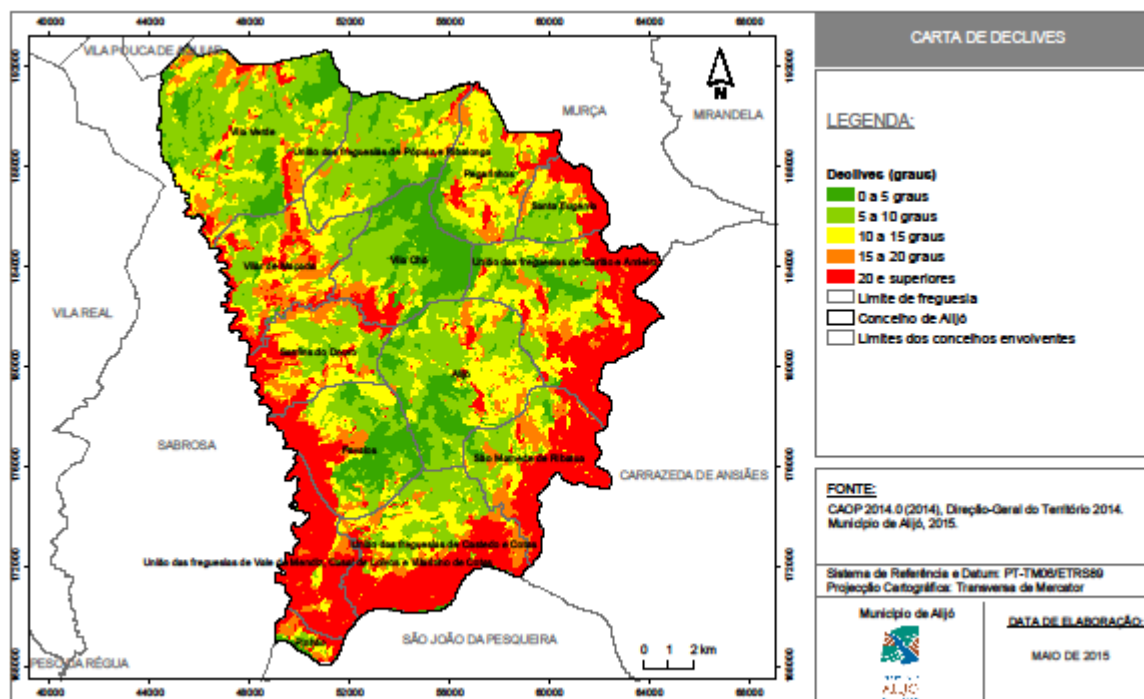
Mapa 5 – Mapa de Declives do Concelho de Alijó
