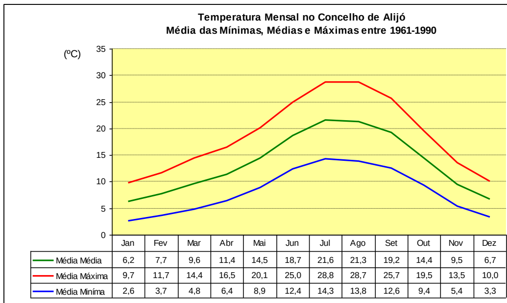
Mapa 8 – Mapa Temperaturas Mensais do Concelho de Alijó
