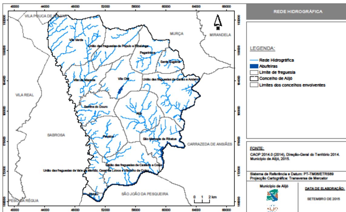
Mapa 7 – Mapa Hidrográfico do Concelho de Alijó
