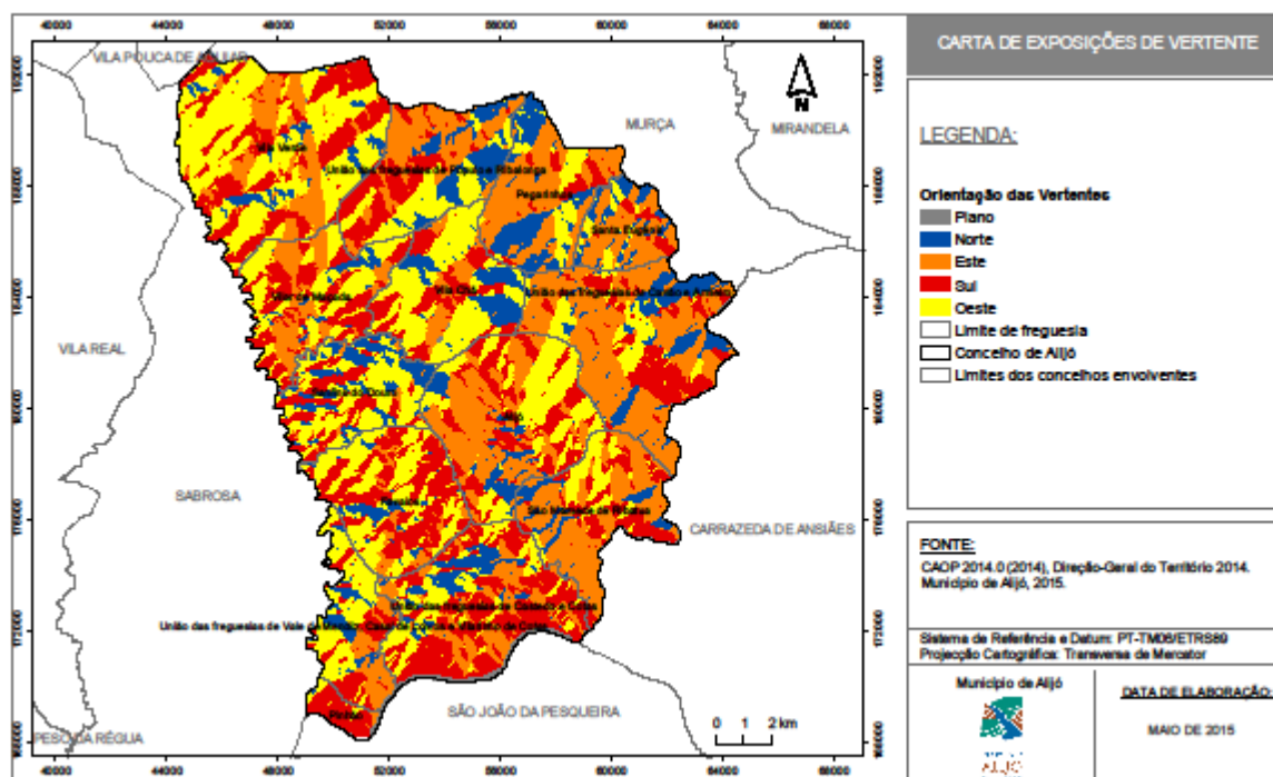
Mapa 6 – Mapa de Exposição do Concelho de Alijó
