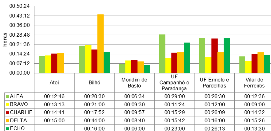
Gráfico 4 - Valor médio por freguesia do tempo de chegada para a 1.ª intervenção, nas fase de perigo
