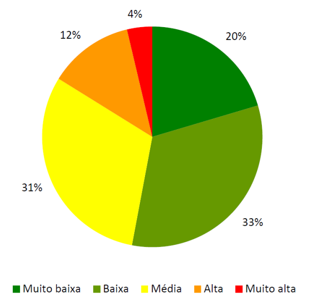
Gráfico 2- Área ocupada por classe de perigosidade
