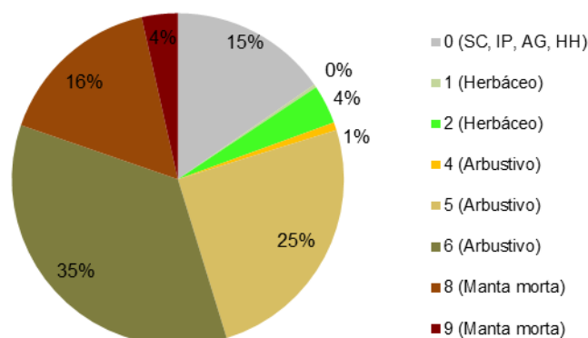
Gráfico 1- Modelos de combustível (%)
