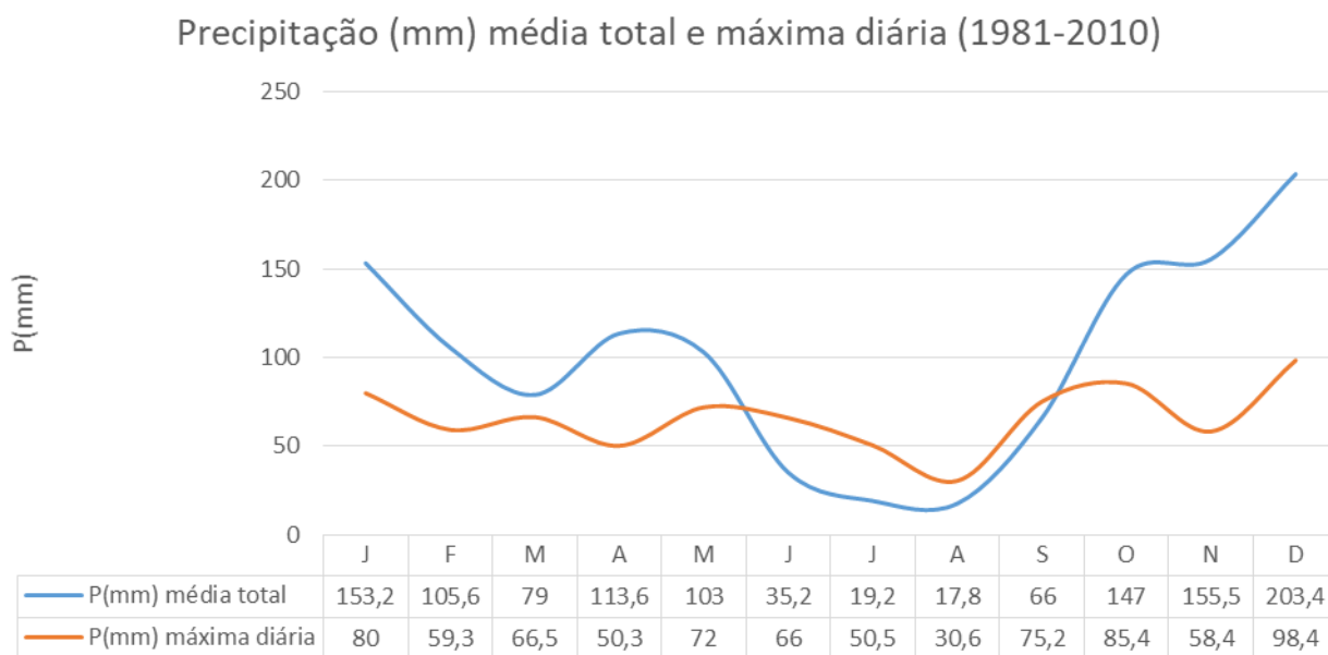
Gráfico 9– Precipitação (mm) média total e máxima diária (1981-2010)
