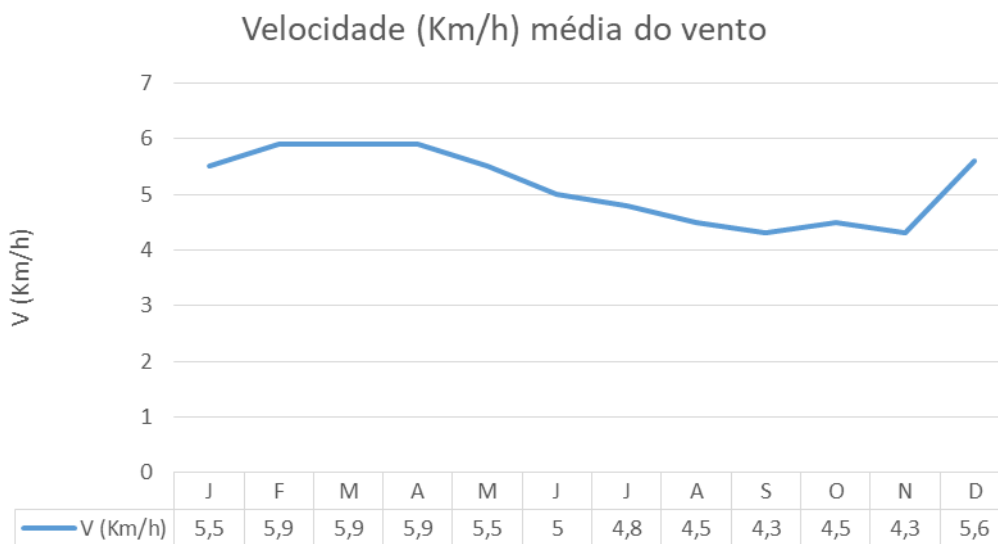
Gráfico 12 - Velocidade média (Km/h) do vento (1971-2000)
