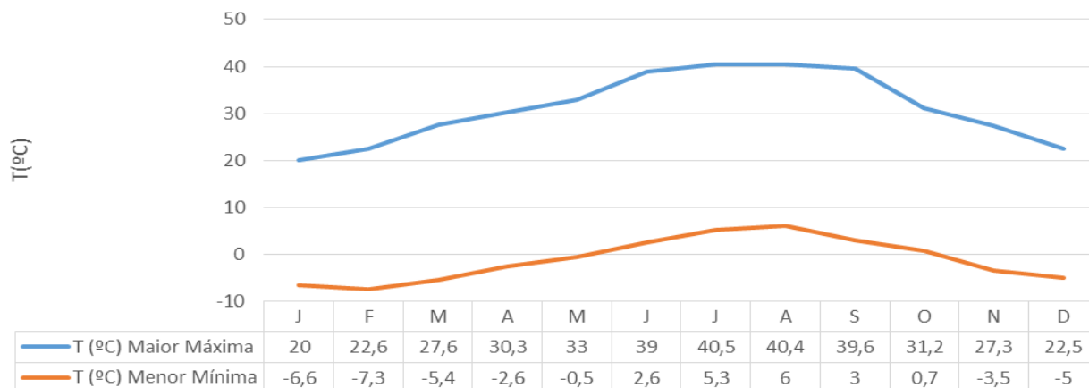
Gráfico 6– Valores extremos de temperatura (°C) (maior máxima e menor mínima) (1981-2010)
