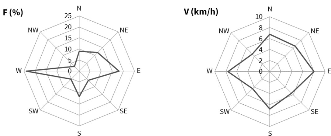
Gráfico 10 – Frequência (%) e velocidade do vento (rumo)
