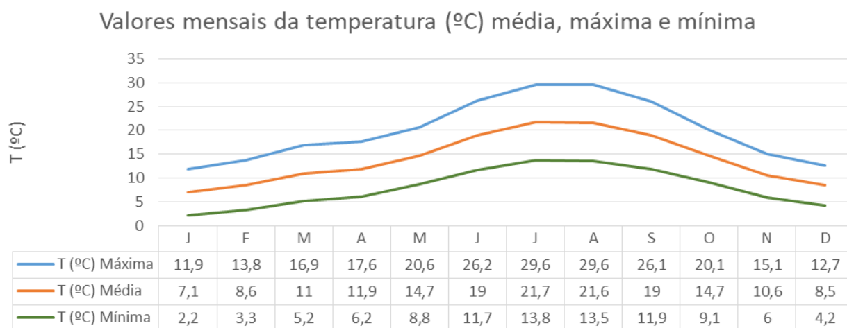
Gráfico 5– Valores médios mensais da temperatura média, máxima e mínima (1981-2010)
