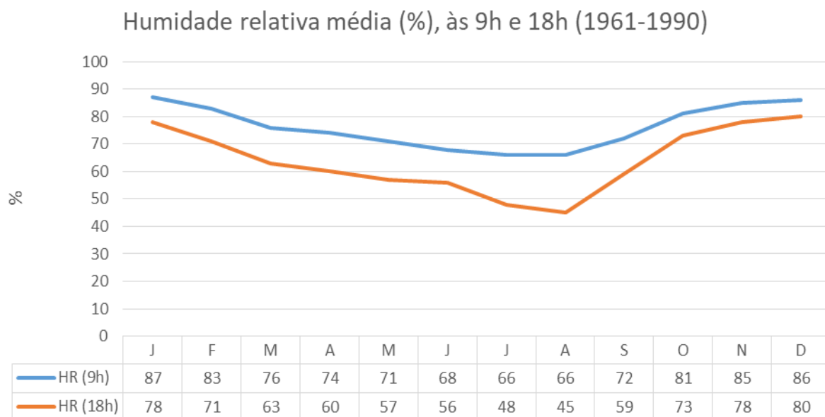
Gráfico 7– Humidade relativa do ar às 9h e 18h (1961-1990)
