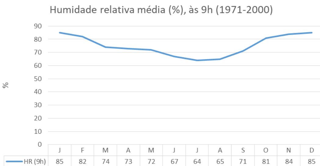
Gráfico 8– Humidade relativa média (%), às 9h (1971-2000)
