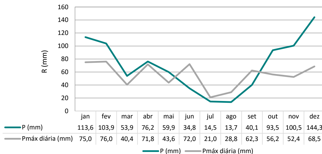
Gráfico 5: Valores mensais da precipitação e máximas diárias
